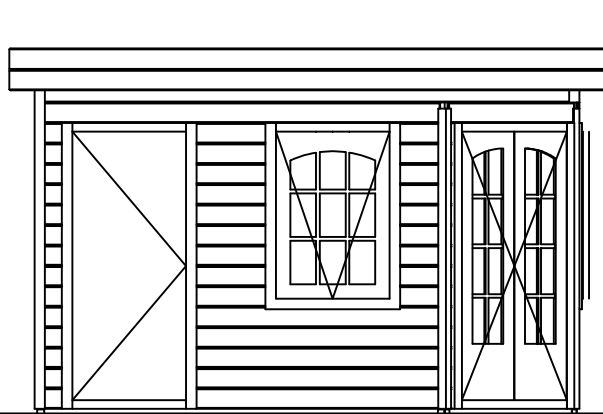
Voorraanzicht / Front view / Vorderansicht
