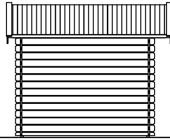
(L) Zijaanzicht / Side view / Seiten ansicht
