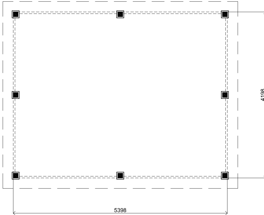
Plattegrond / Plan
